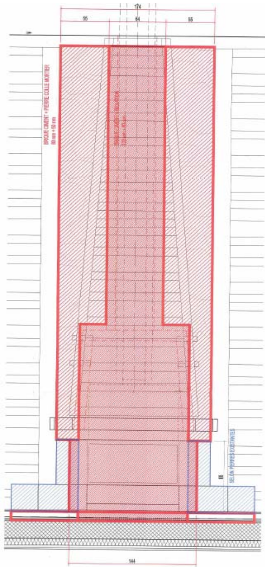
Coupe verticale
