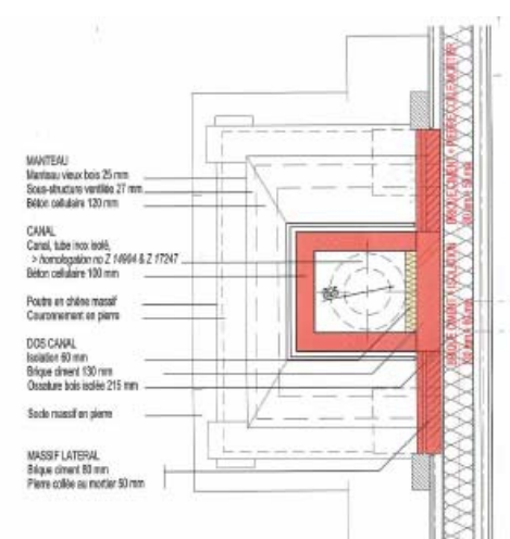
PLAN AU NIVEAU DE L'ETAGE 1/20
