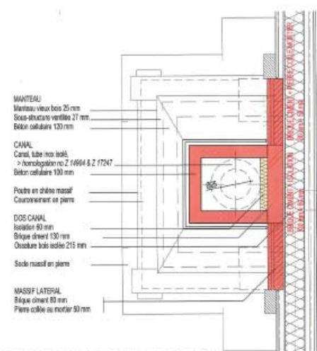
PLAN AU NIVEAU DE L'ETAGE 1/20
