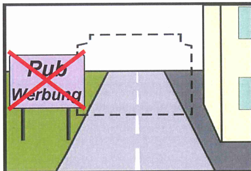
Placé dans le gabarit d'espace libre de la chaussée (OSR, art. 96, al. 2, lettre a)
