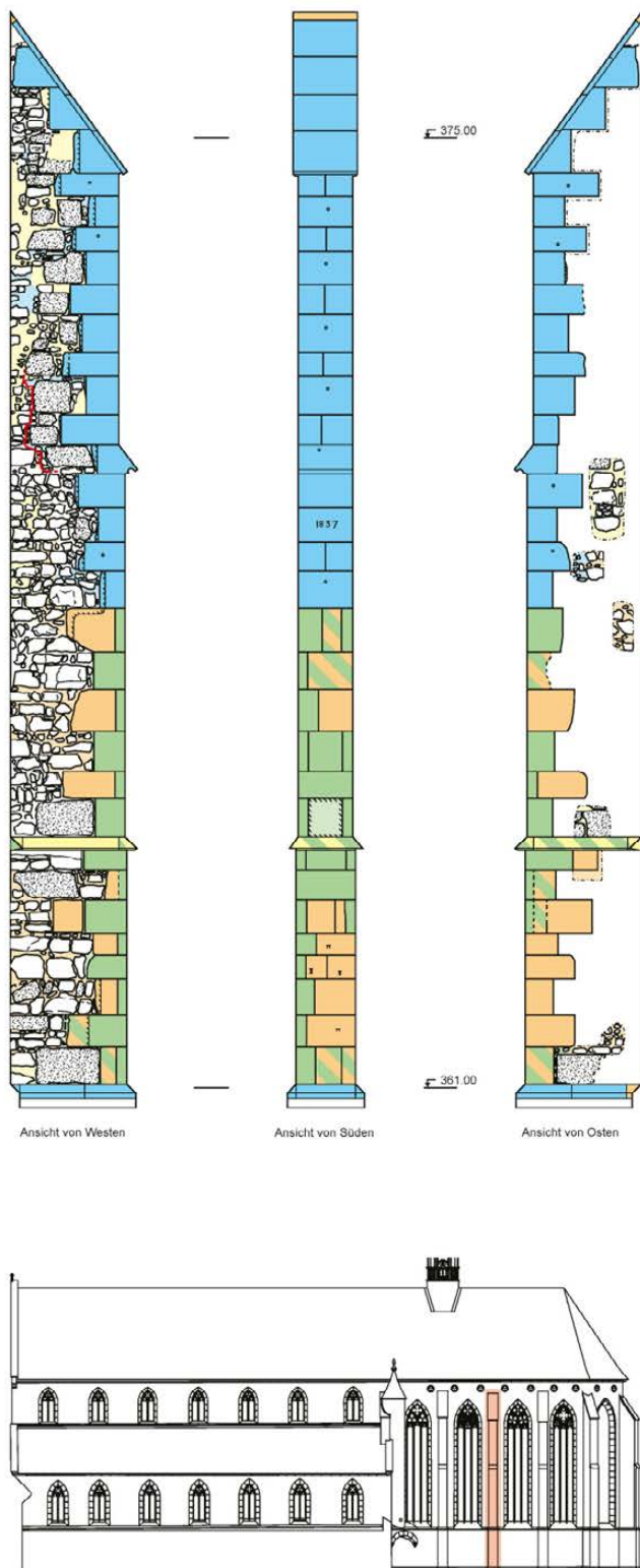
Abb. 75. Windisch AG, Kloster Königsfelden. Umzeichnung des zweiten Strebepfeilers von Westen der Chor-Südseite. Farblich sind der originale Bestand (Steine matt; dazugehöriger Mauermörtel/Mörtelverputz transparent) und die unterschiedlichen Restaurierungskampagnen dargestellt. Orange: Bauzeit 1320–1330. Blau: Ersatz der Sandsteinblöcke durch Muschelkalkblöcke um 1837. Grün: Ersatz der Sandsteinblöcke (bzw. ihrer Häupter) durch Sandsteinplatten um 1892. Gelb: Ersatz der Sandsteinblöcke/Werksteine durch maschinell gefertigte Steine 1984. Plan KAAG.
