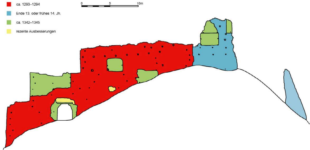
Abb. 72. Seewis im Prättigau GR, Solavers. Südfassade der bestehenden Schildmauer. Vereinfachter Bauphasenplan. AD GR.
