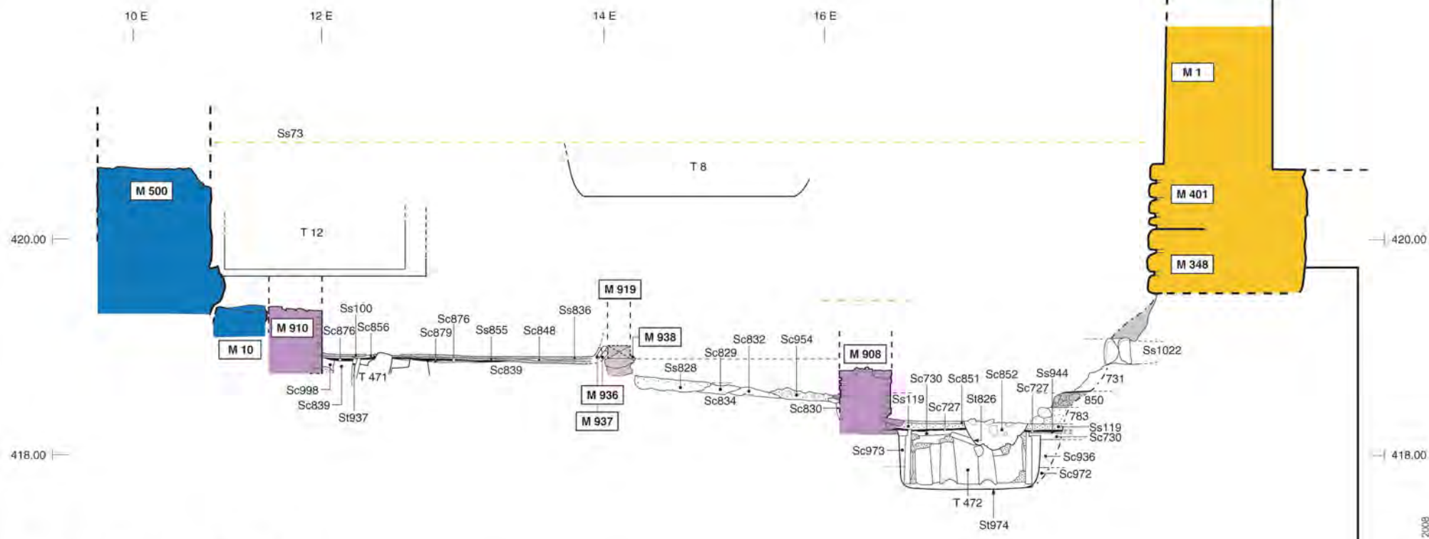
Saint - Maurice, Martolet coupe schématique E-W axe: 16 N
