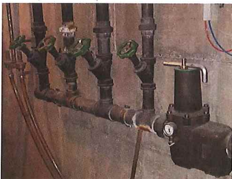
Nourrice d'eau sanitaire
