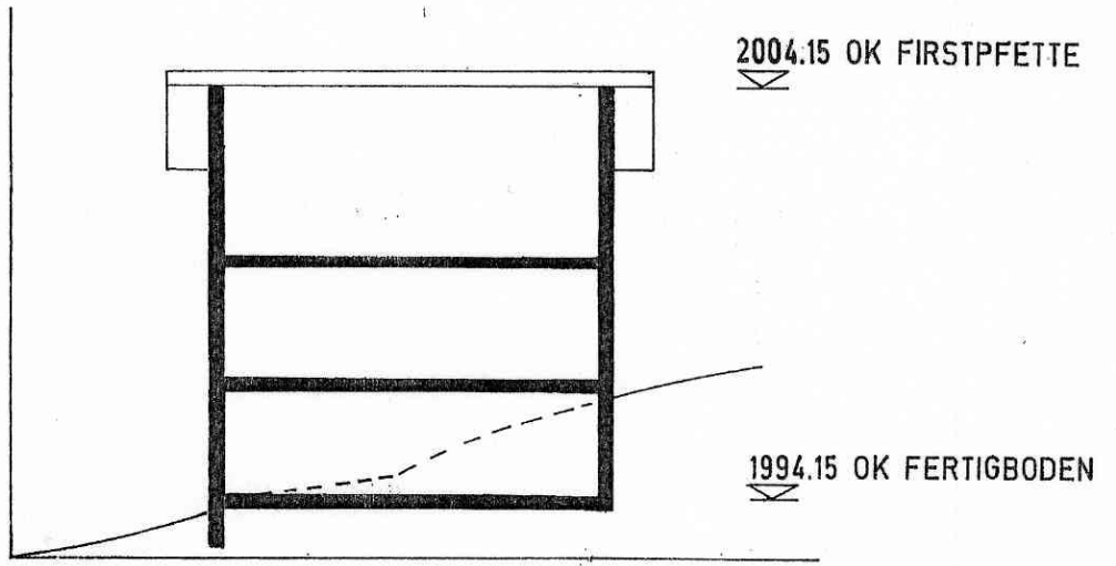
PROFILSCHNITT BREITEN 1
