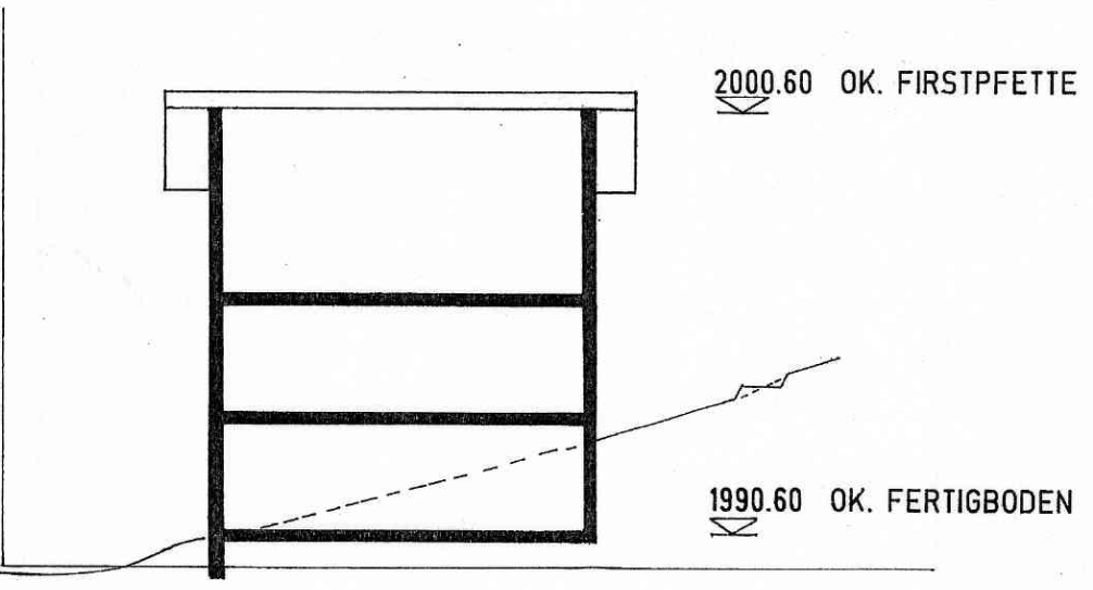
PROFILSCHNITT BREITEN 2
