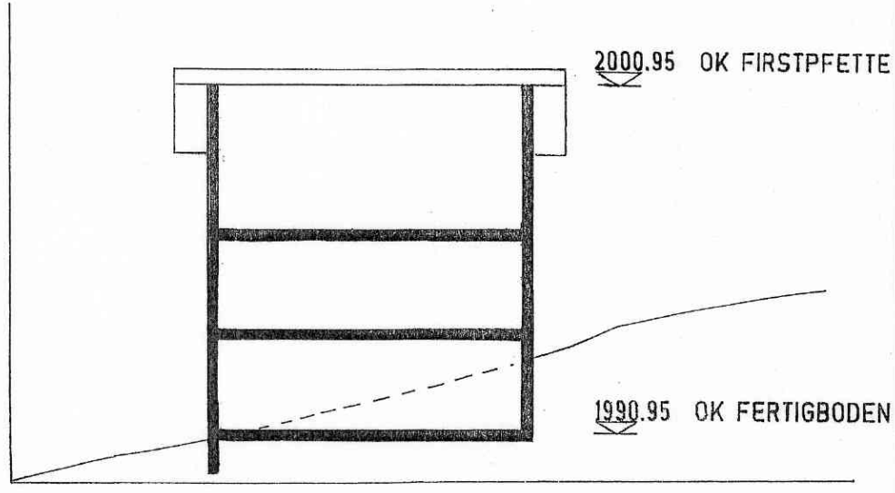
PROFILSCHNITT BREITEN 3
