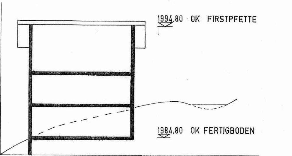
PROFILSCHNITT BREITEN 8
