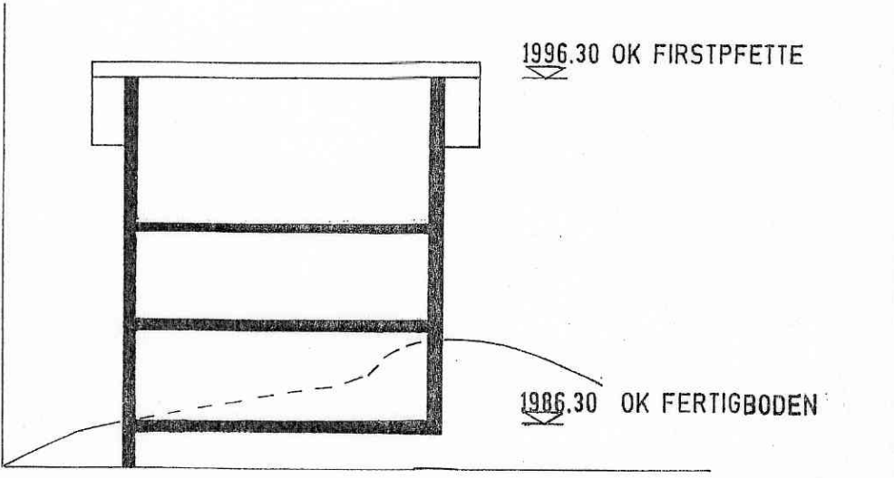
PROFILSCHNITT BREITEN 5
