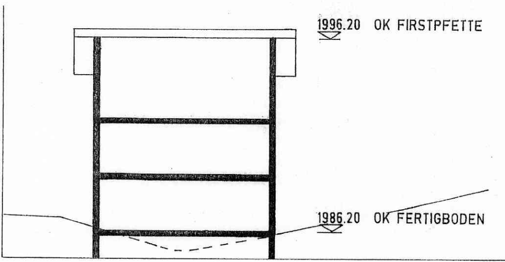
PROFILSCHNITT BREITEN 7
