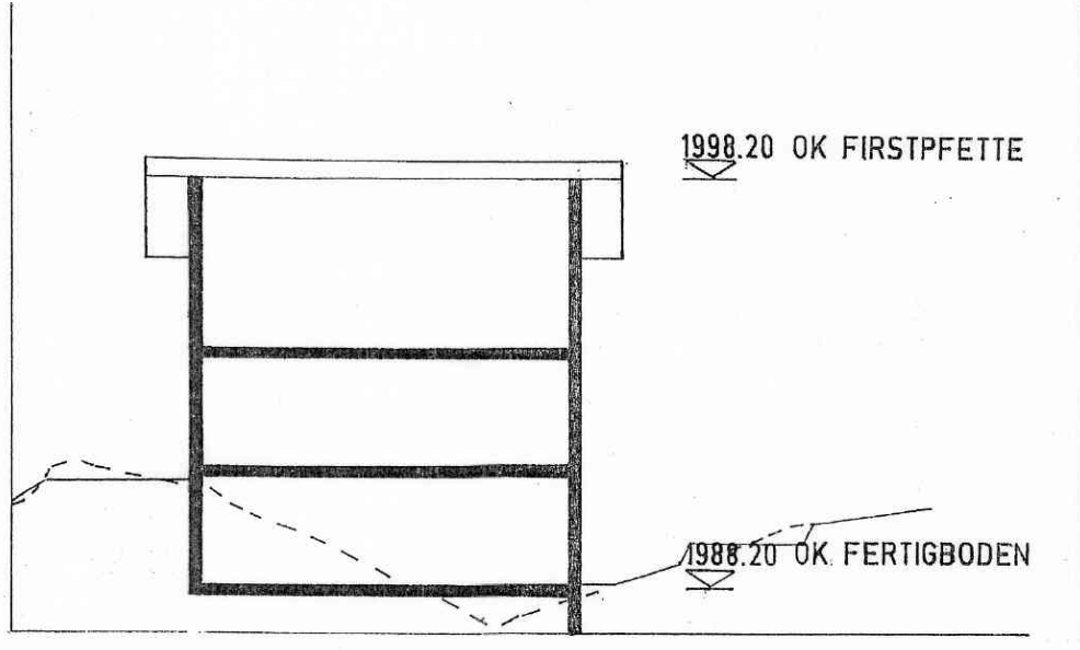
PROFILSCHNITT BREITEN 4
