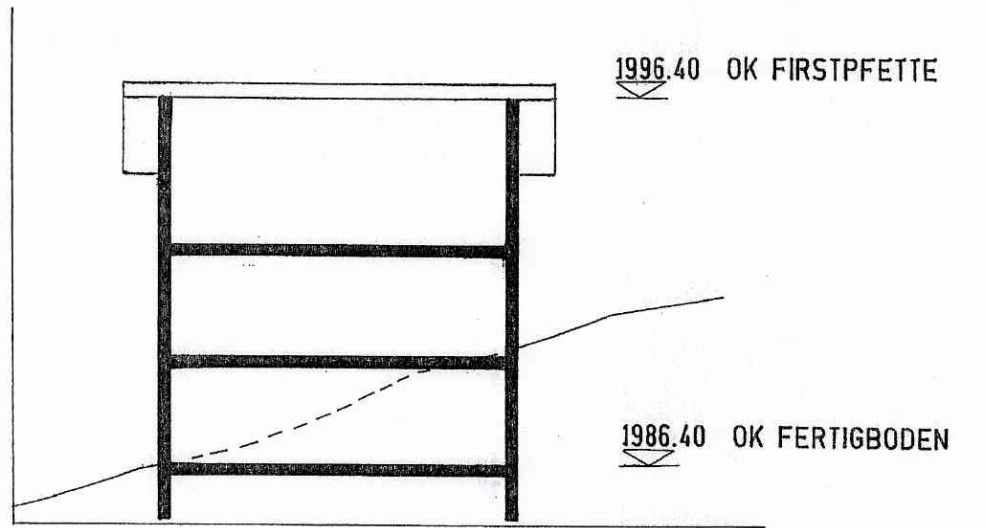
PROFILSCHNITT BREITEN 6
