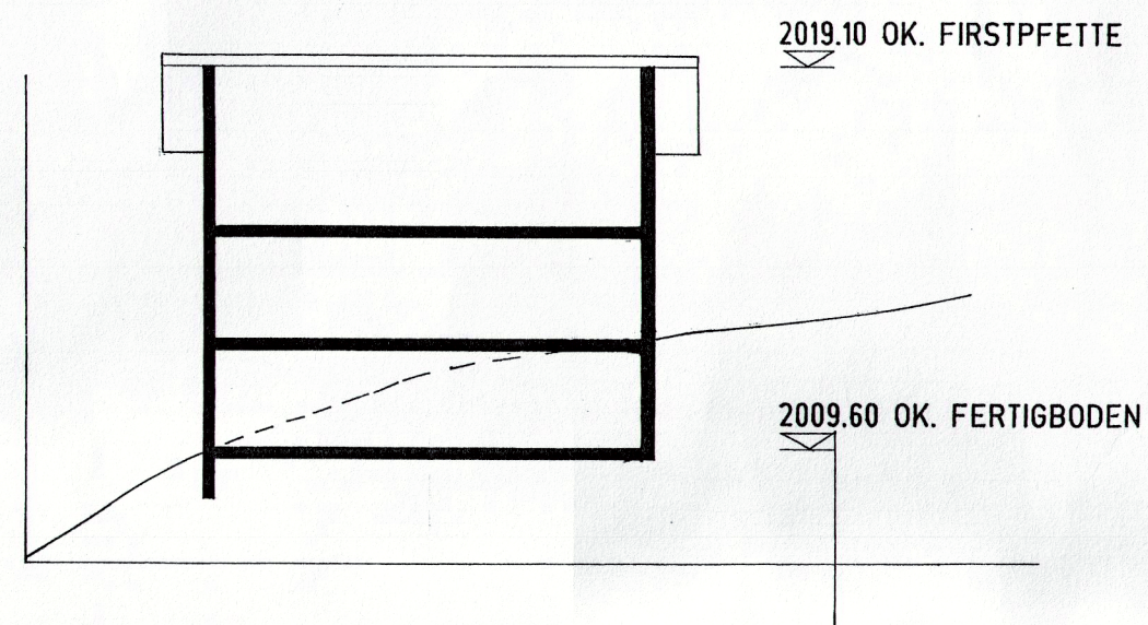
PROFILSCHNITT DOMO 1
