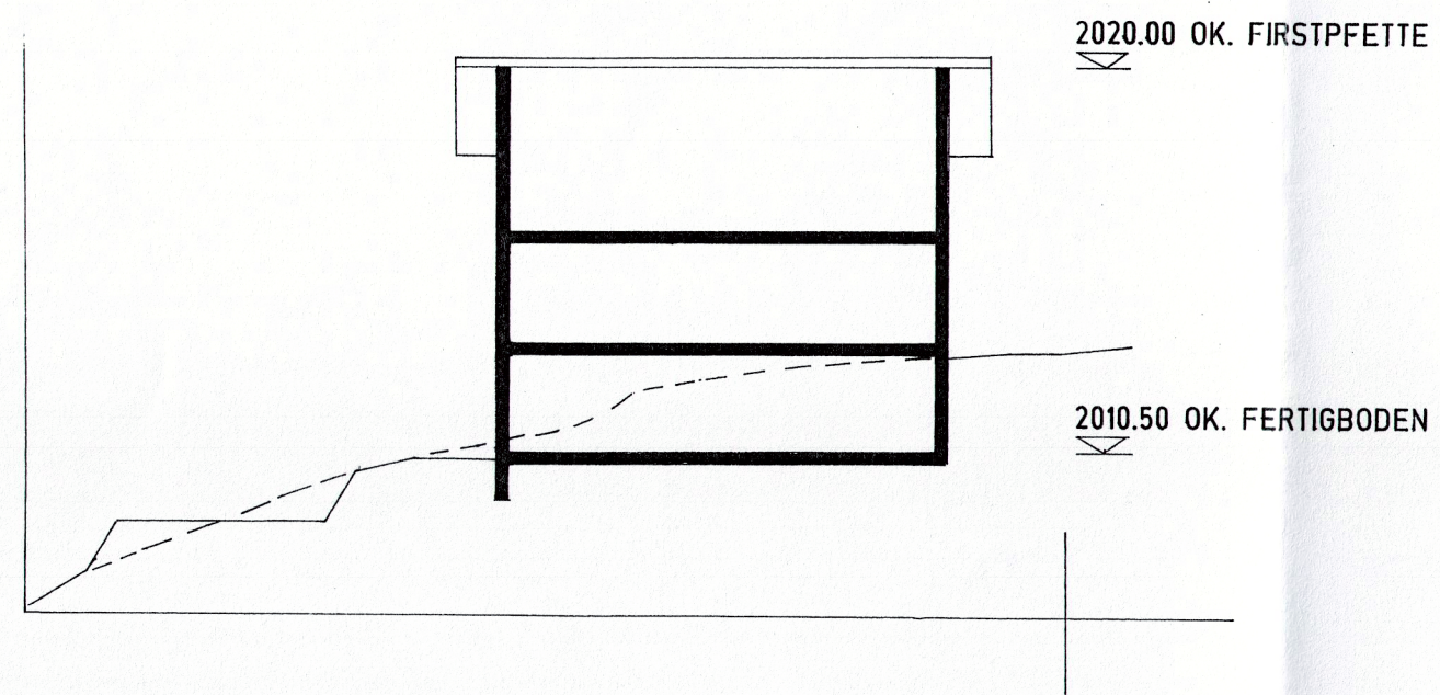
PROFILSCHNITT DOMO 3
