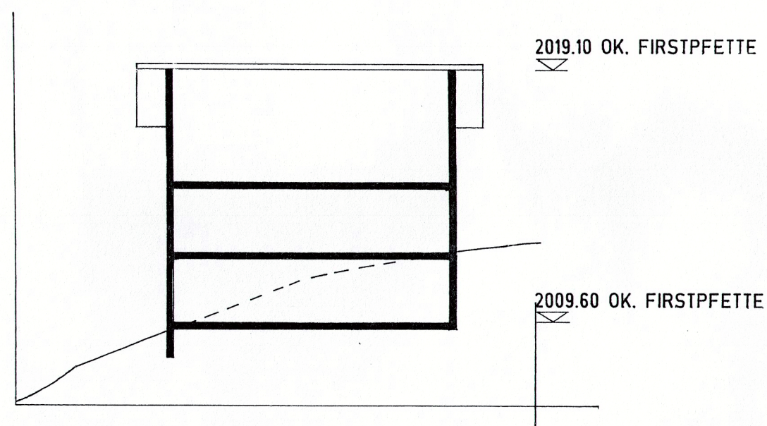
PROFILSCHNITT DOMO 2
