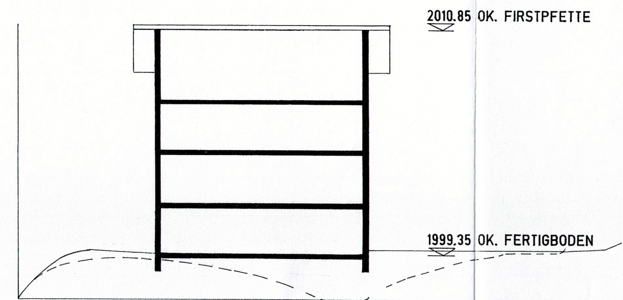
PROFILSCHNITT DOMO 6
