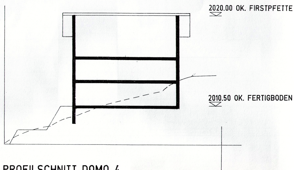
PROFILSCHNITT DOMO 4
