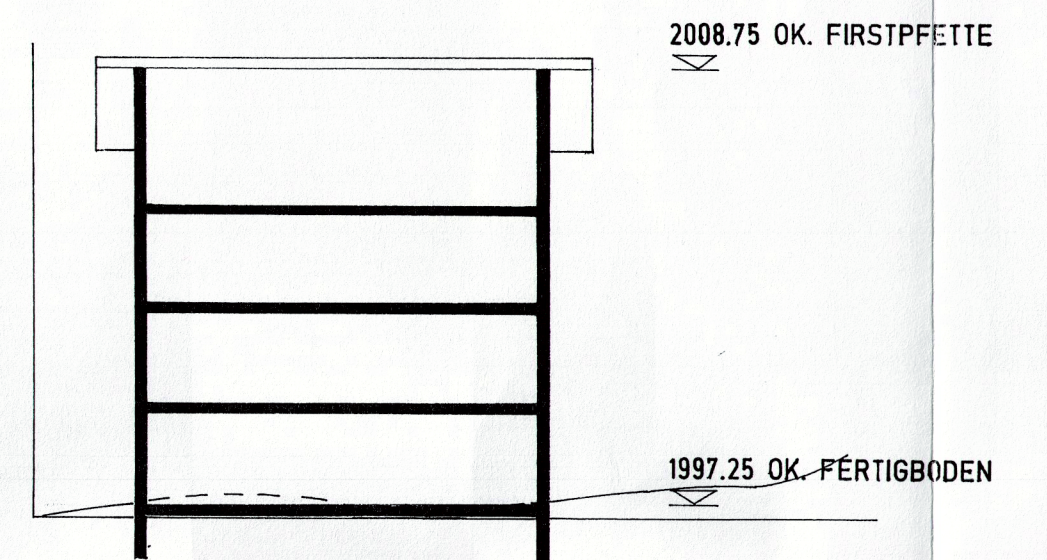
PROFILSCHNITT DOMO 7
