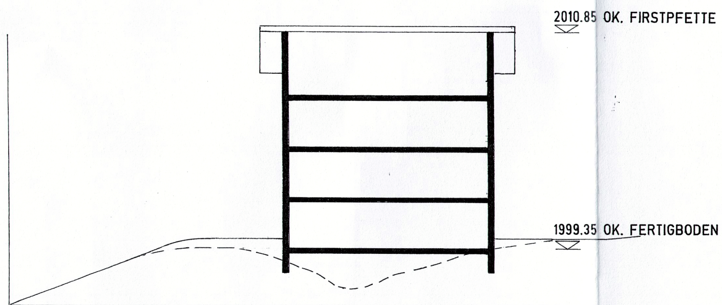
PROFILSCHNITT DOMO 5
