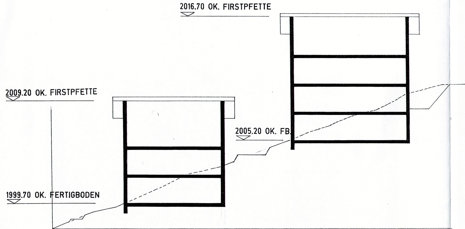
PROFILSCHNITT BODMEN 2 UND 3
