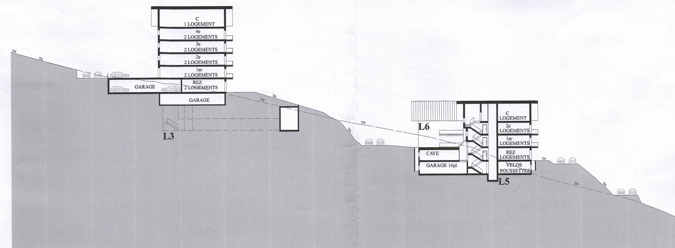
Coupe 4-4, ech. : 1/500
