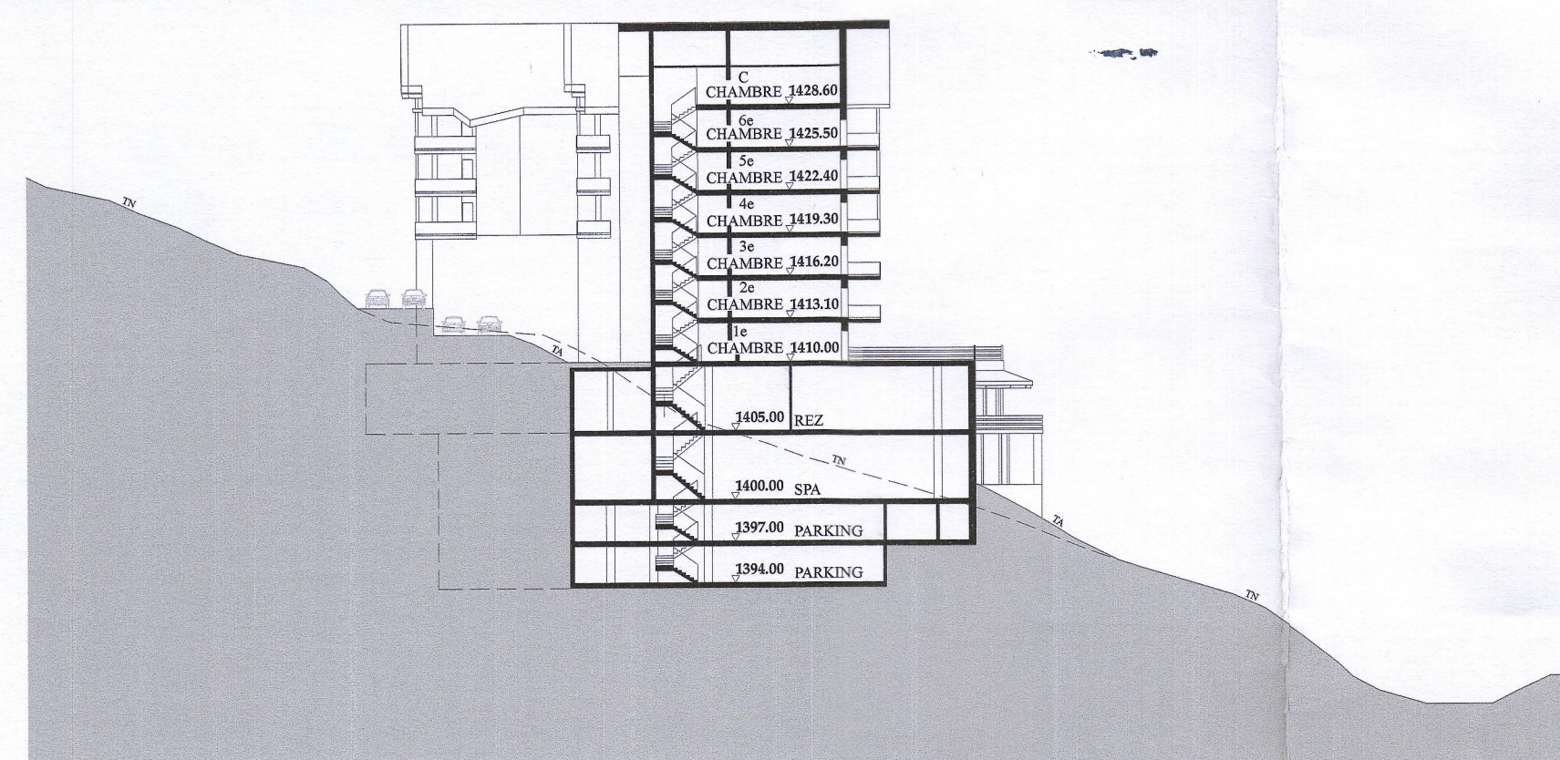
Coupe 3-3, ech. : 1/500
