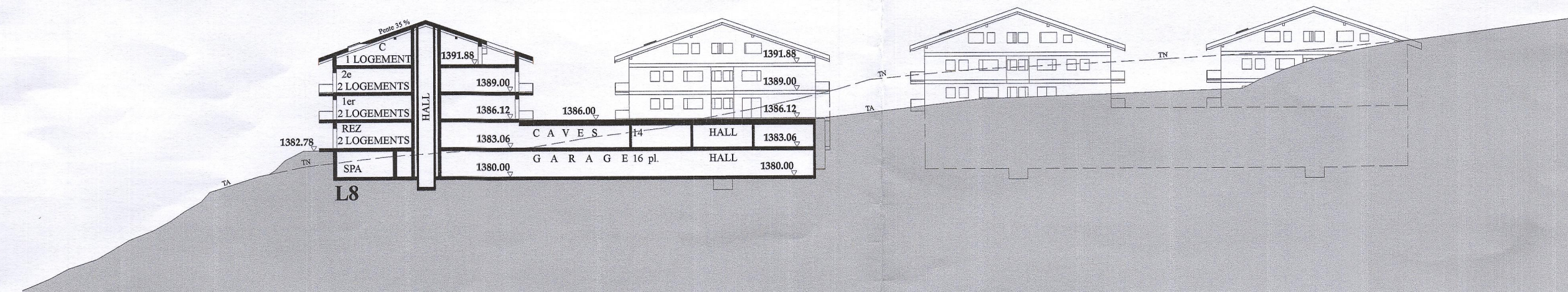
Coupe 2-2, ech. : 1/500
