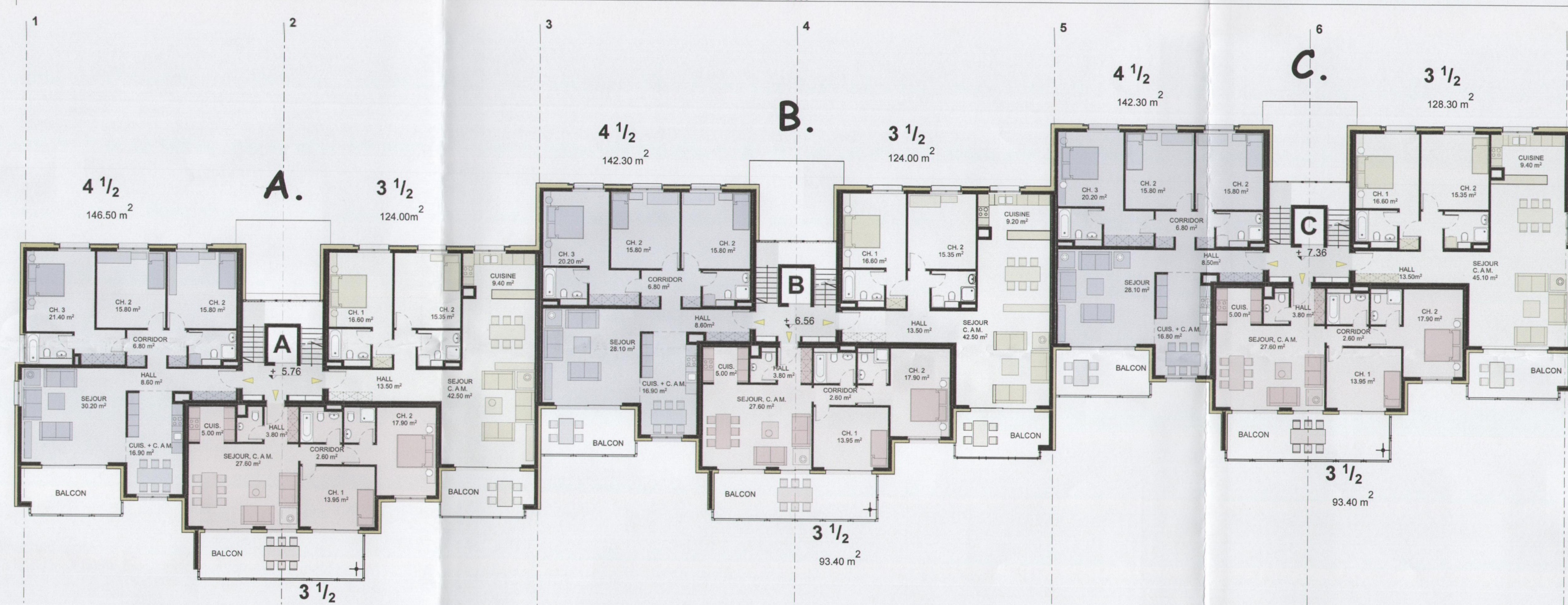
2 ème ETAGE
