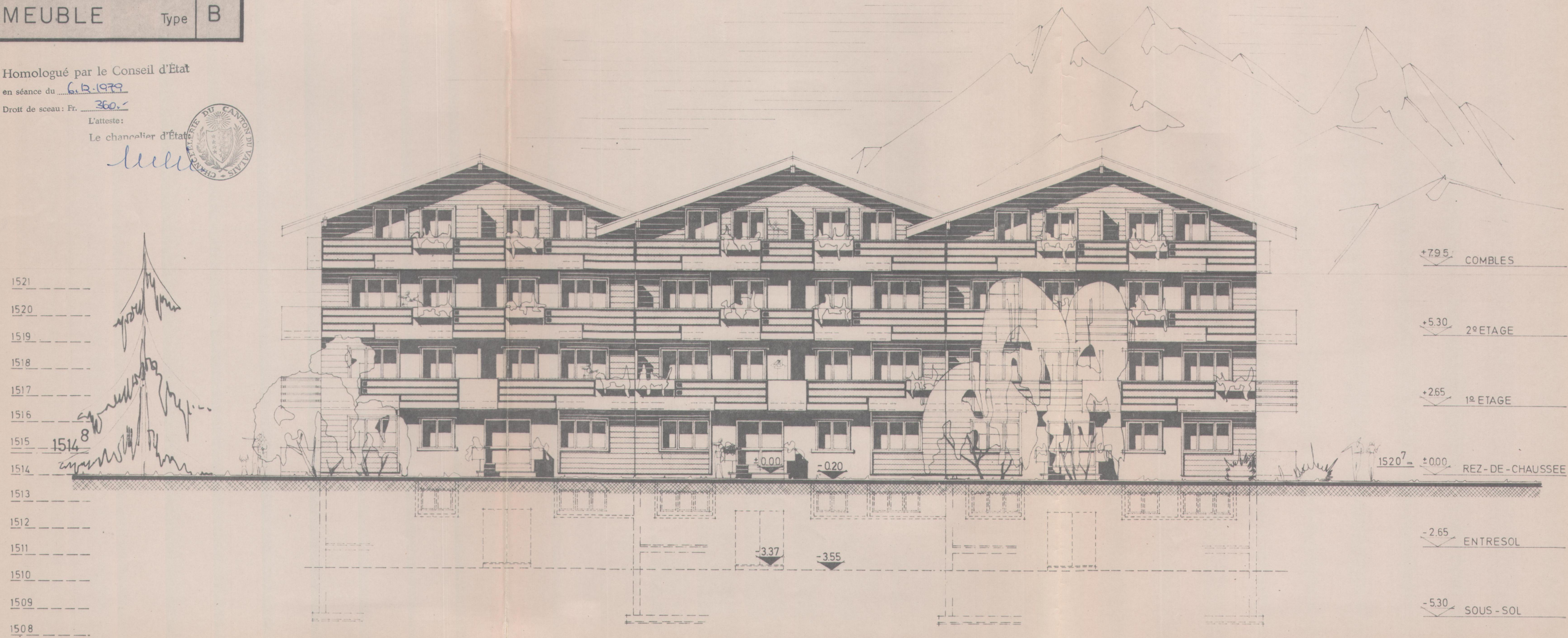
FACADE SUD-OUEST
