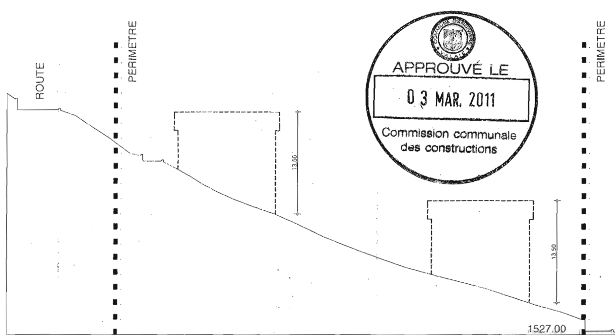
COUPE C-C
