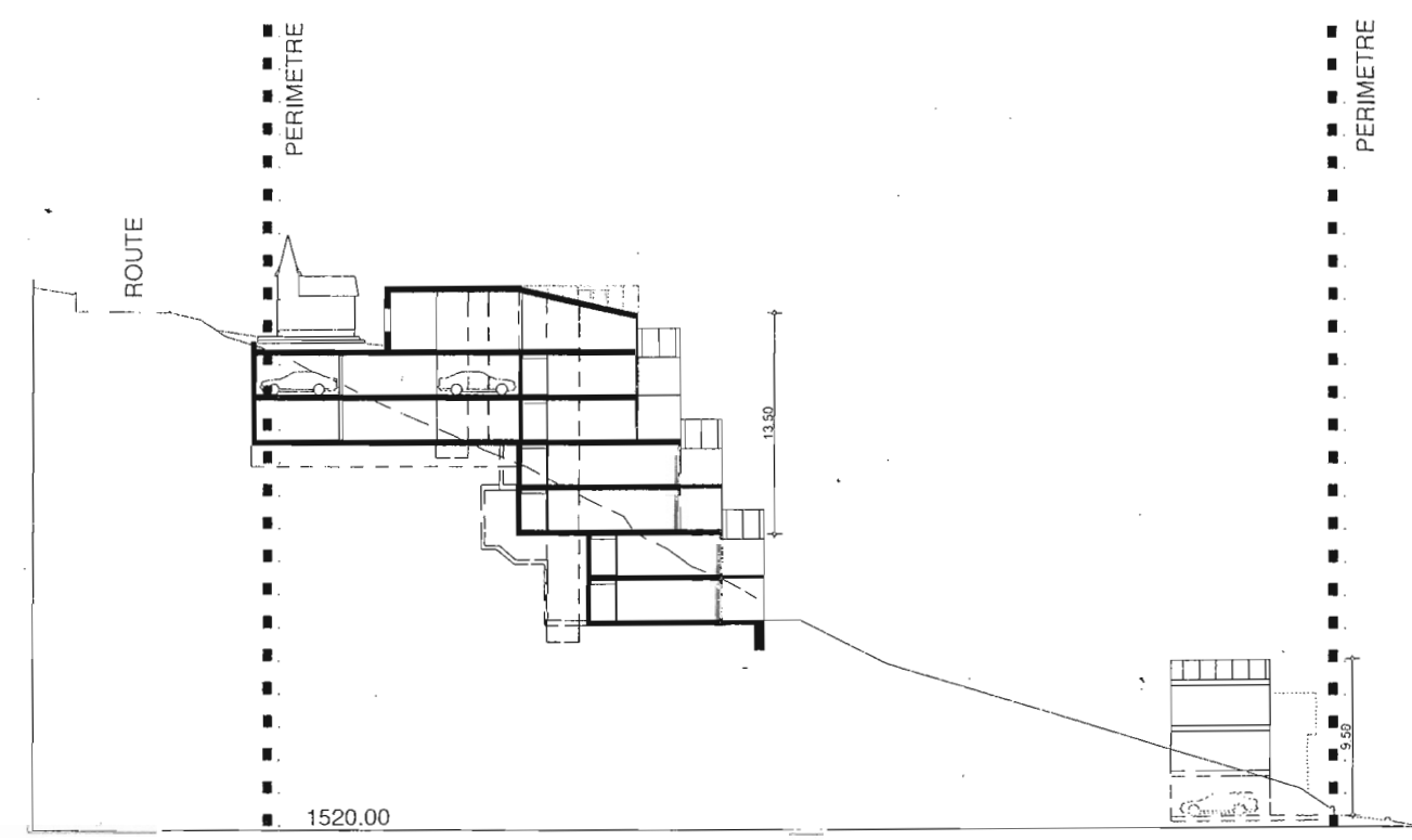
COUPE E-E
