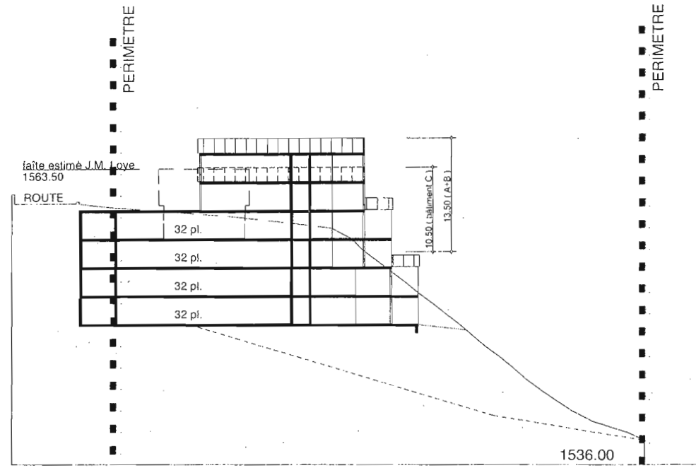
COUPE A-A
