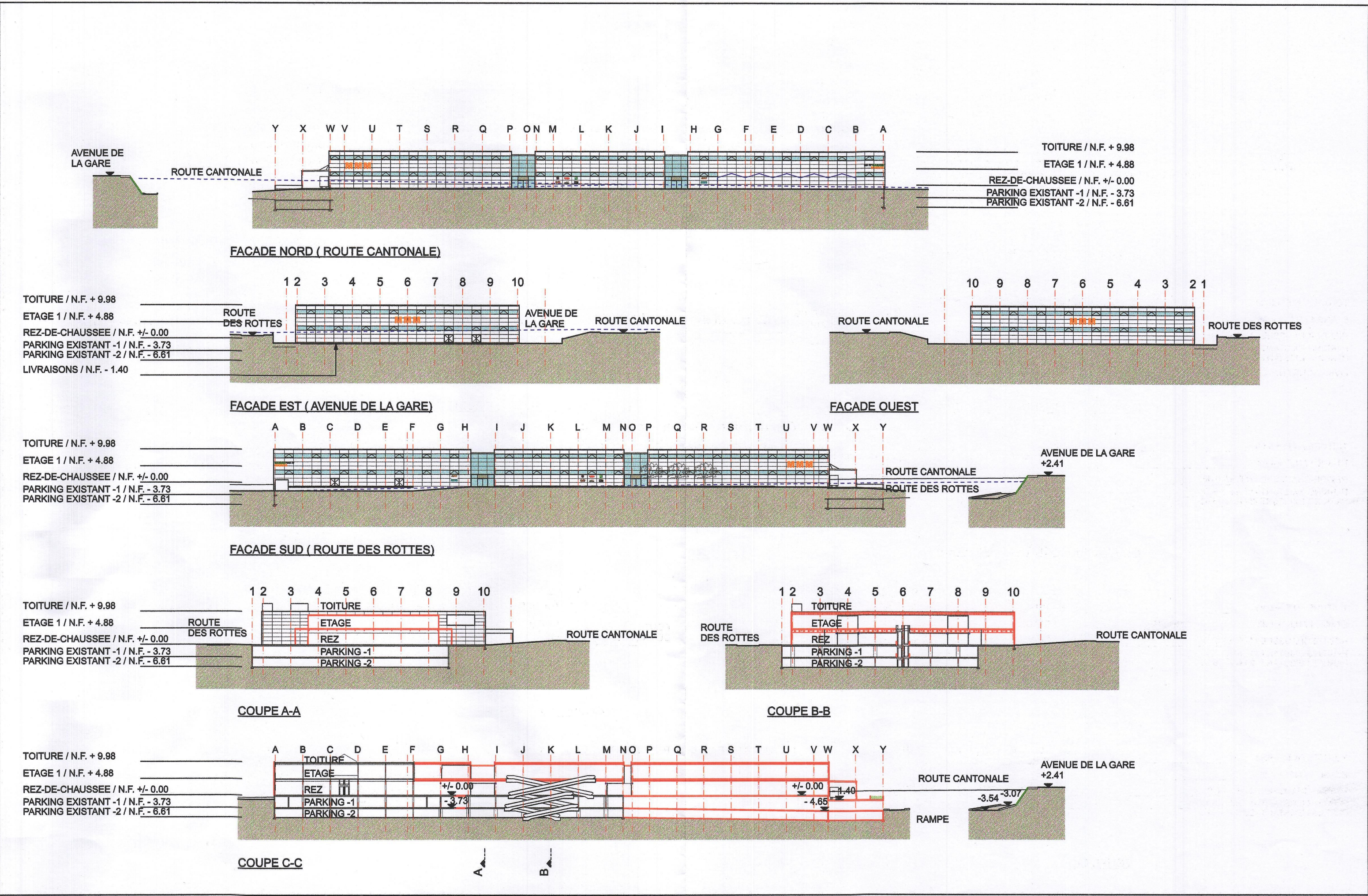
COUPES + FACADES
