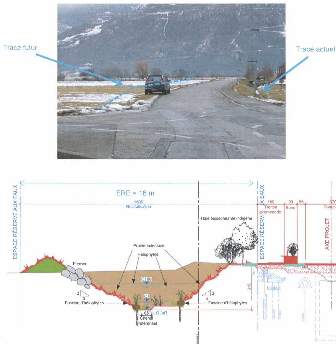
Figure 14: Tronçon 6025 – PLA01, état actuel (en-haut) et coupe type du projet d'aménagement des torrents Ouest [2] avec ERE (en bas)
