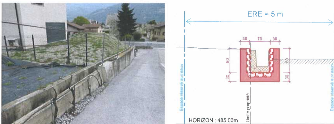
Figure 17: Tronçon 6025 – PLA04, état actuel (à gauche) et coupe type du projet d'aménagement des torrents Ouest [2] avec ERE (à droite)
