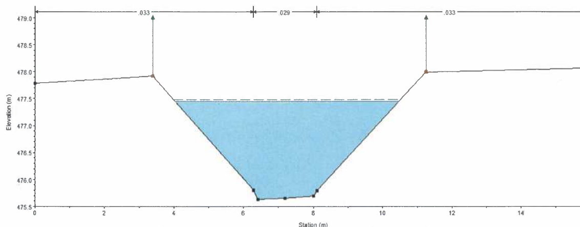
Figure 7: Relevé de section du canal du Couchant
