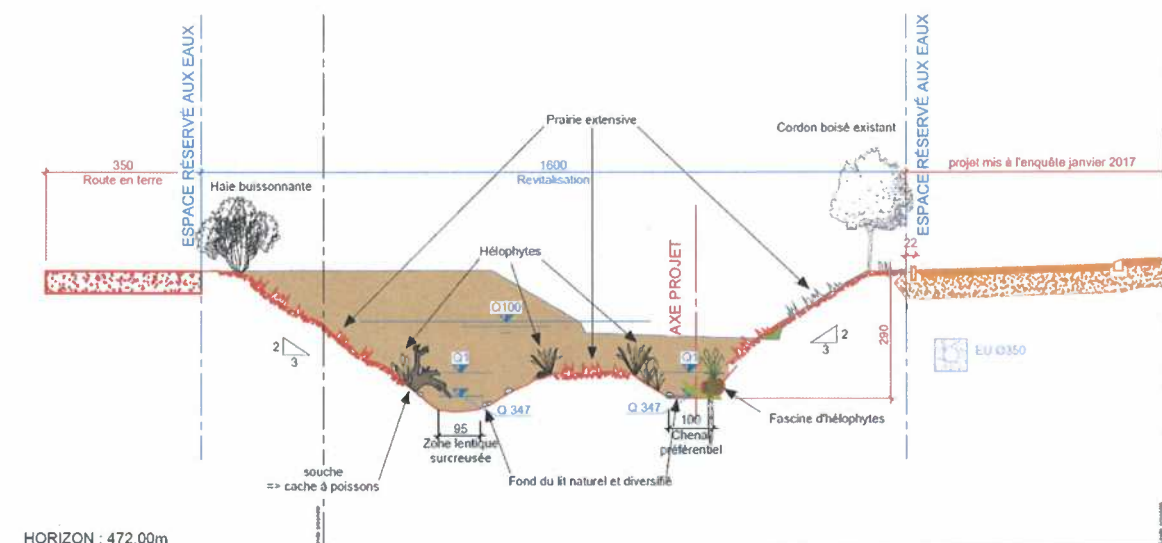
Figure 13 : Coupe type du projet de revitalisation et d'aménagement du canal du Couchant, avec l'ERE, le projet routier en rive droite et la route en terre en rive gauche.
