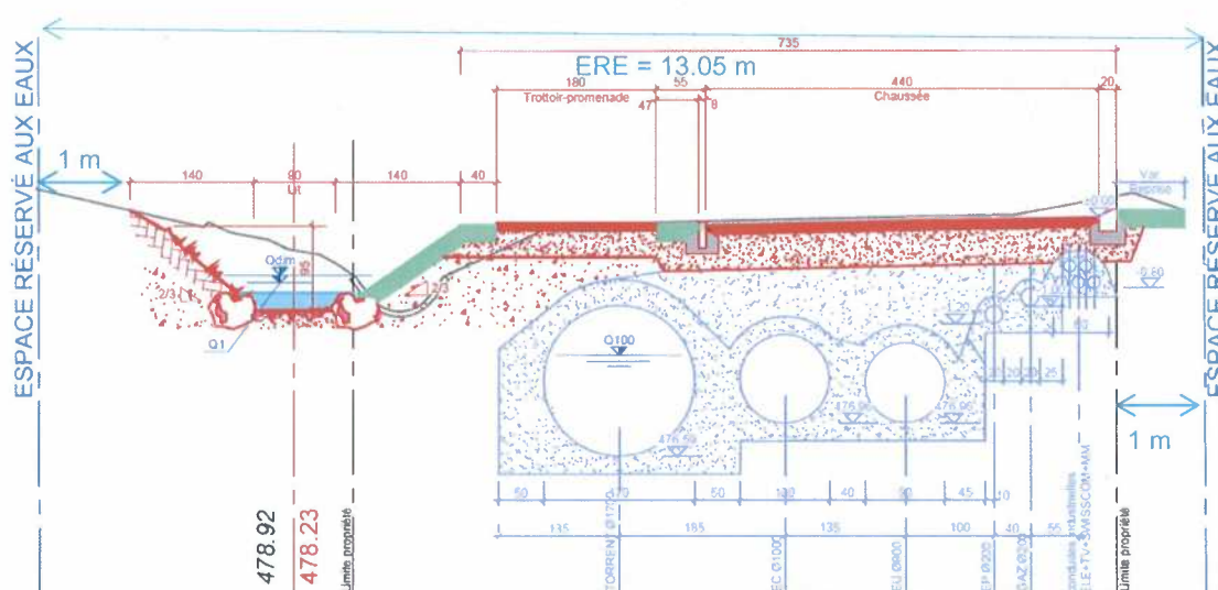
Figure 15: Tronçon 6025 – PLA02, état actuel (en-haut) et coupe type du projet d'aménagement des torrents Ouest [2] avec ERE (en bas)
