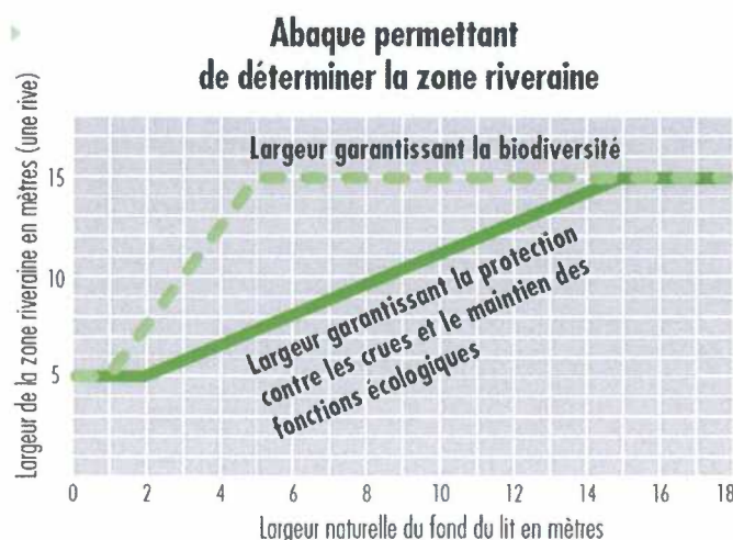
Figure 12: Abaque servant à réserver l'espace des cours d'eau de moins de 15 m de largeur.
