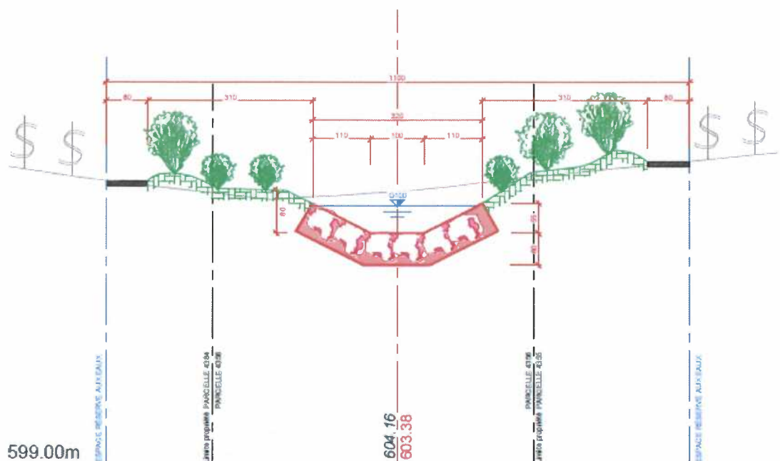
Coupe type du projet d'aménagement des torrents Ouest [2] avec ERE en amont du dépôt
