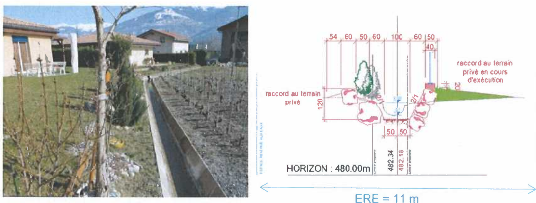
Figure 10: Tronçon 6025 – CRE03, état actuel (à gauche) et coupe type du projet d'aménagement des torrents Ouest [2] avec ERE (à droite)
