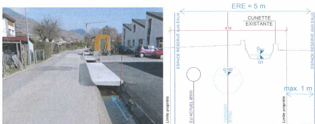
Figure 8: Tronçon 6025 – CRE01, état actuel (à gauche) et coupe type du projet d'aménagement des torrents Ouest [2] avec ERE (à droite)
