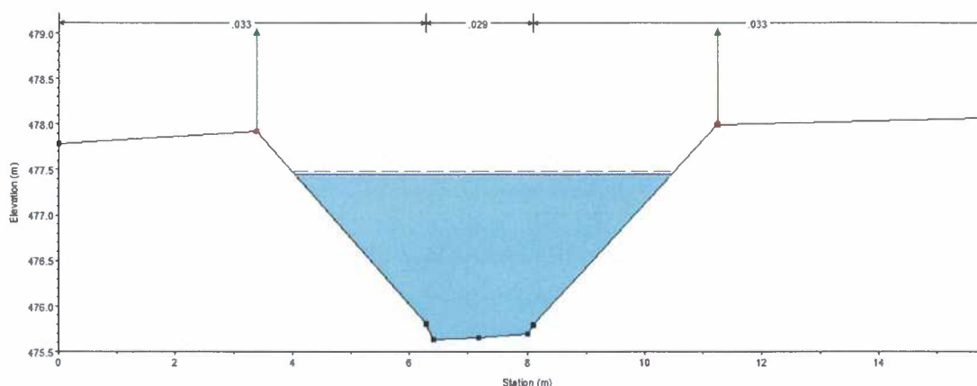
Figure 4: Relevé de section du canal du Couchant
