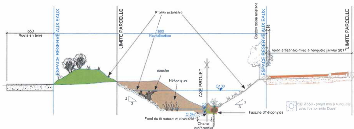
Figure 6 : Coupe type du projet de revitalisation et d'aménagement du canal du Couchant, avec l'ERE, le projet routier en rive droite et la route en terre en rive gauche.
