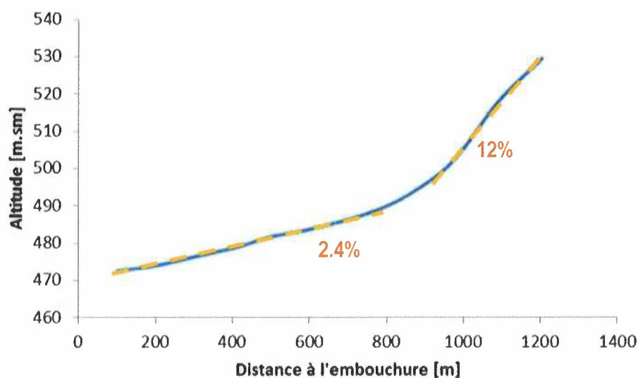
Figure 3: Profil en long de la Losentze, avec détail de la pente moyenne
