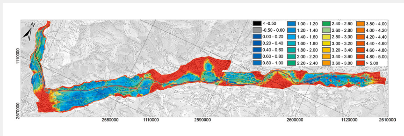
Fig. 5 Épaisseur moyenne de la zone non saturée en mètre représentative du mois de février calculée pour la période de référence 1976-2017 (secteur Sierrre-Évionnaz).
